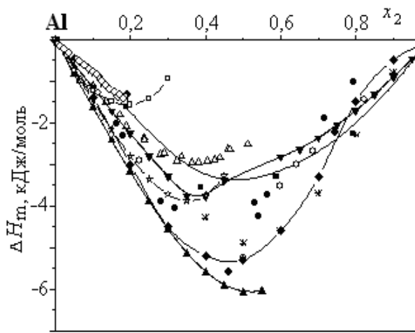
Рис. 1. Інтегральні ентальпії змішування розплавів Al – Si:
