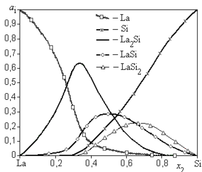
Рис. 5. Мольні частки (і активності) компонентів та асоціатів у розплавах La – Si за 1820 К
