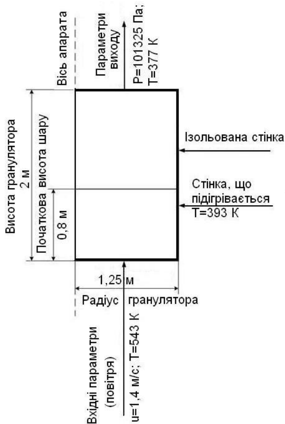
Рис. 1. Параметри моделювання апарата з псевдозрідженим шаром
