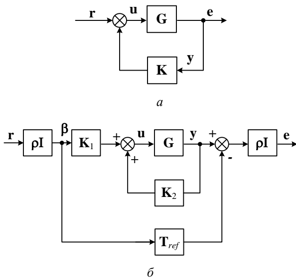
Рис. 1. Структури систем із регуляторами:
