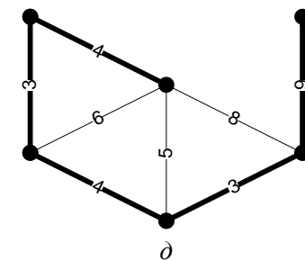
Рис. 4. Алгоритм Борувки: a – початковий стан. (Підграф A складається з n вершин і порожньої множини ребер); b – для кожної компоненти зв'язності (вершини) знаходимо безпечне ребро (позначено стрілками); v – додаємо ребра до підграфу A ; z – для кожної компоненти зв'язності знаходимо безпечні ребра (відмічені стрілками); d – додаємо ребра до підграфу A . (Мінімальне зв'язне дерево T побудовано.)
