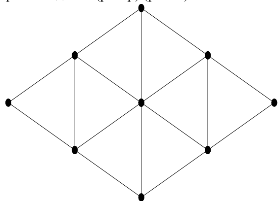
Рис. 2. Граф G
