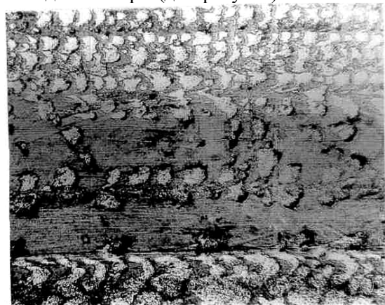
Трибоструктура на поверхні електролітичного хрому (темні ділянки) після тертя по сталі 45 у гідрорідині АМГ-10, \times 200
