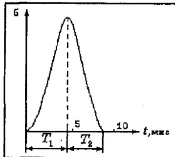
Рис.3. Імпульс розвантаження, який генерується при утворенні тріщини довжиною 17 мм: v_p/v_{зв} = 0,5 ( v_p – швидкість зростання тріщини; v_{зв} – швидкість звуку); T_1, T_2 – тривалість переднього та заднього фронтів зміни напруг
