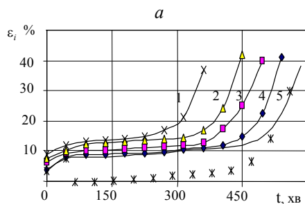
Рис. 1. Ізотермічна повзучість титанового сплаву VT20:
