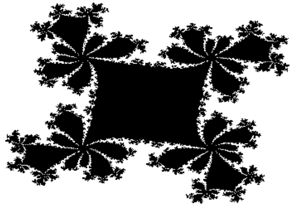
Fig. 1. Fractal set images with different parameters: a) C=(0.590; 0.420) , N=3 ; b) C=(0.589; 0.420) , N=3 ; c) C=(0.590; 0.420) , N=4 ; d) C=(0.610; 0.450) , N=4
