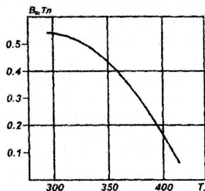
Рис. 1. Зависимость намагниченности магнитных покрытий от температуры
