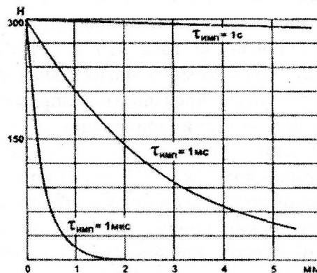
Рис. 2. Графики изменения амплитуды напряженности магнитного поля в зависимости от толщины корпуса НЖМД
