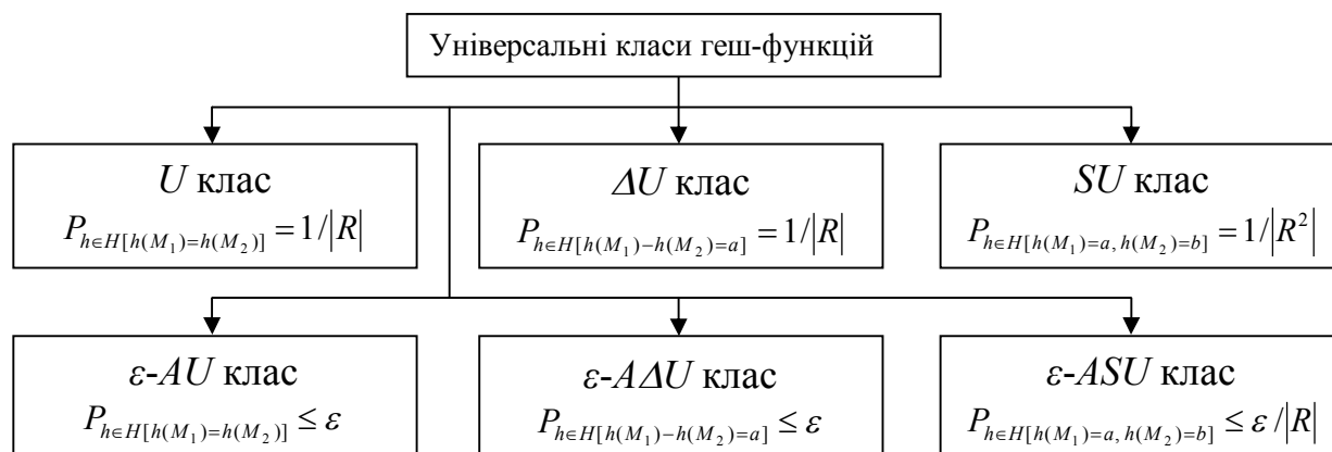
Рис. 5. Класифікація універсальних класів гешування
