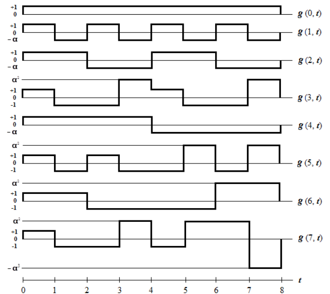
Рис. 1. Базисные ФЗС восьмого порядка
