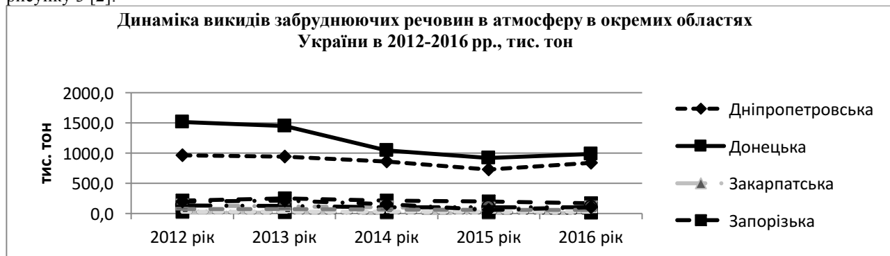
Рис. 3 Динаміка викидів забруднюючих речовин в атмосферу в окремих областях України в 2012-2016 рр., тис. Тон
