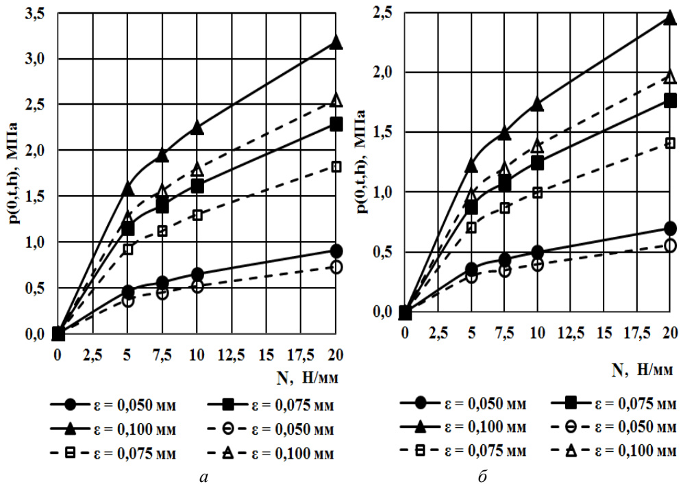
Рис. 5. Трибологічні тиски у напрямній при зміні навантаження та зношуванні втулки: а – композит Моглайс; б – ДК6
