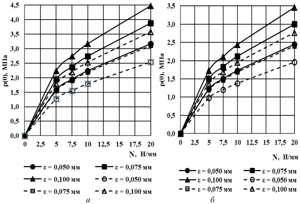
Рис. 4. Залежність p(0) від N : а – композит Моглайс; б – ДК6
