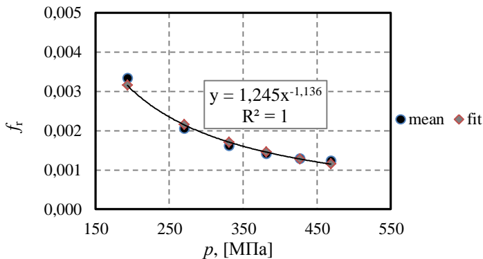
Рис. 7. Усереднена апроксимована залежність коефіцієнту тертя кочення від контактний тиску
