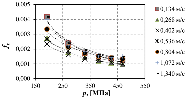
Рис. 6. Залежність коефіцієнту тертя коченню від величини контактного тиску за різних колових швидкостей
