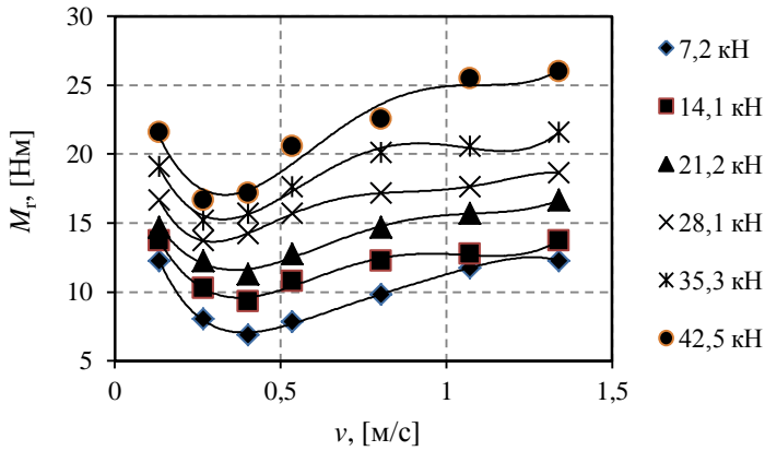
Рис. 4. Залежність моменту тертя кочення від колової швидкості та контактної сили
