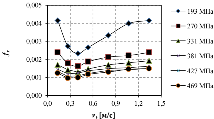
Рис. 5. Залежності коефіцієнту тертя кочення від колової швидкості за різних значень контактної сили
