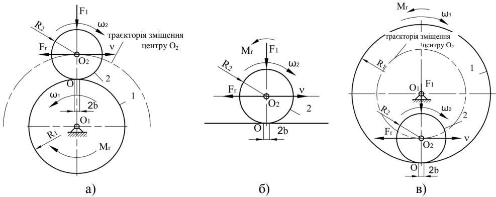
Рис. 1. Типові кінематичні схеми процесу кочення циліндричного ролика: а – по зовнішній циліндричній поверхні, б – по плоскій поверхні
