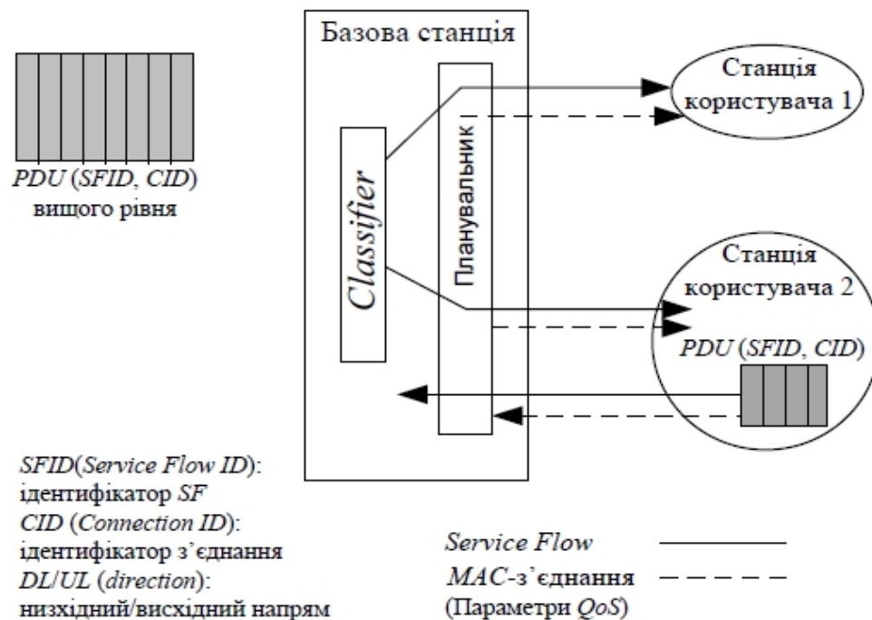
Рис. 1 Підтримка QoS в мережі WiMAX
