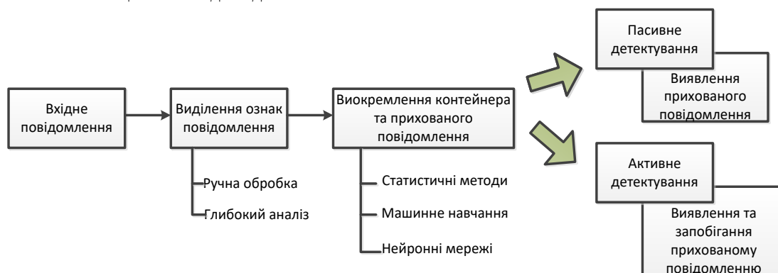
Рис. 2 Загальний алгоритм процесу стегоаналізу повідомлення
