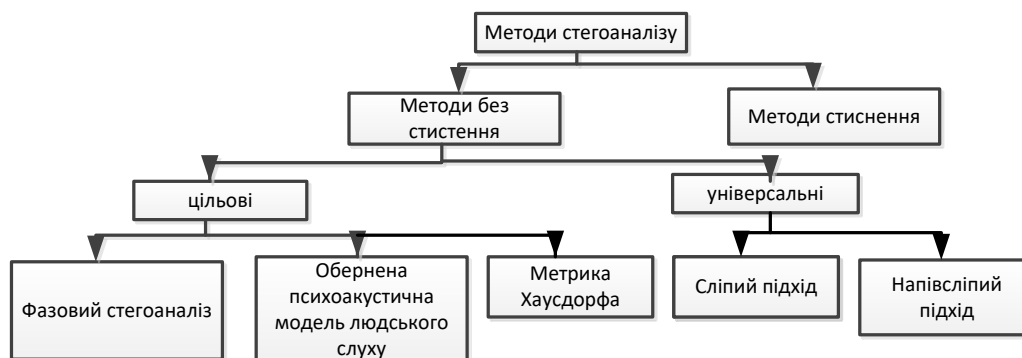
Рис. 1 Загальна класифікація методів стегоаналізу аудіосигналів
