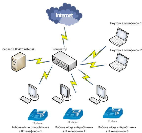
Рис. 2. Схема організації IP телефонії Asterisk
