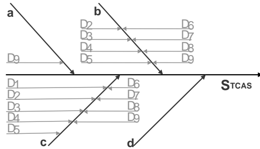
Рис. 3. Причинно-наслідкова діаграма Ісікави для підсистеми S_{TCAS}
