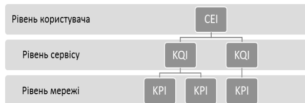
Рис. 1. Рівні оцінки якості функціонування стільникової мережі зв'язку
