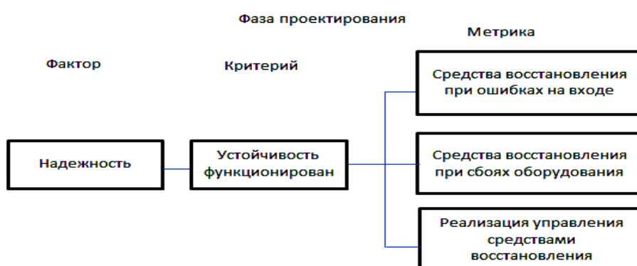
Рис.3 Взаимосвязь факторов, критериев и метрик фазы проектирования качества ПС
