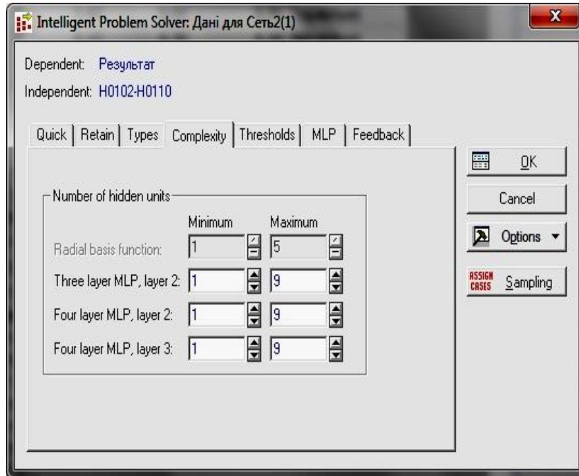
Рис. 6 Вкладка «Сложность» («Complexity») мастера решений
