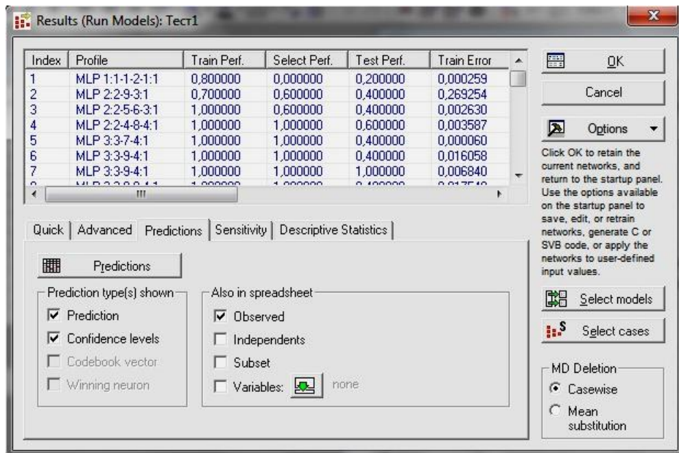
Рис.7. Результаты, характеризующие обученную нейронную сеть
