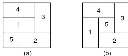
Рис. 1 Приклади простих флорплєнів: а) безрозрізний; б) розрізний [4]
