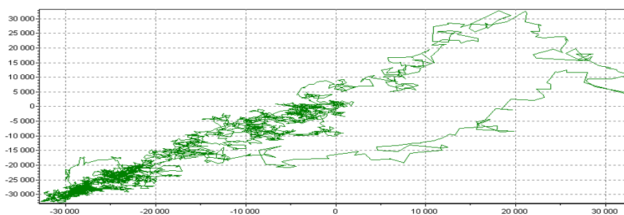
Рис. 3. Фазовий простір ЧР цін на нафту з 20.05.1987 по 20.04.2011 рр.
