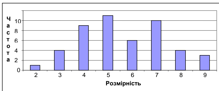
Рис.5. Частота N(L) появи квазіциклів розмірності L ЧР цін на нафту
