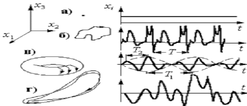
Рис. 1. Приклади характерних множин у фазовому просторі систем з неперервним часом і часових реалізацій рухів, яким вони відповідають
