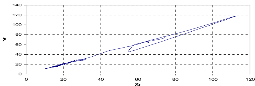
Рис.6. Траєкторія еволюції центрів квазіциклів ЧР
