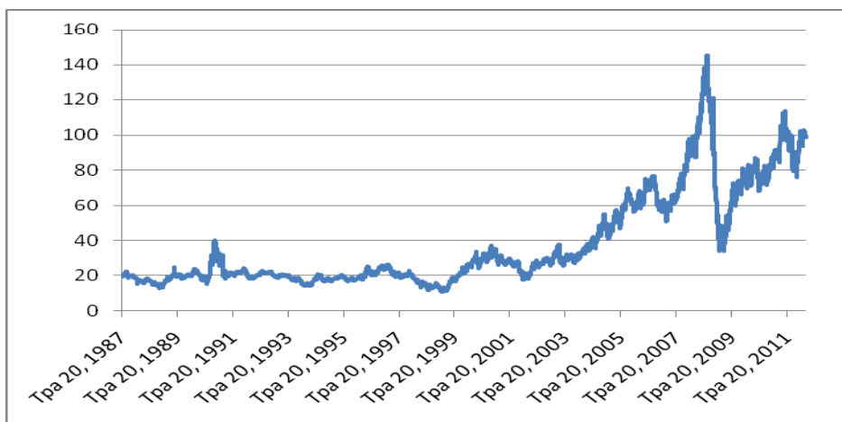
Рис.2. Денні ціни на нафту марки Brent
