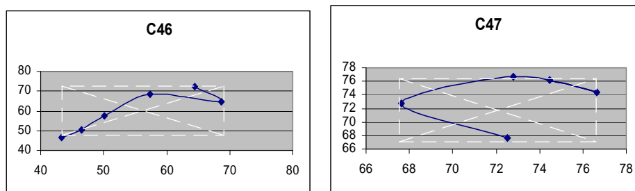
Рис. 4. Фрагмент розкладання на квазіцикли ЧР цін на нафту за травень – липень 2010 р.
