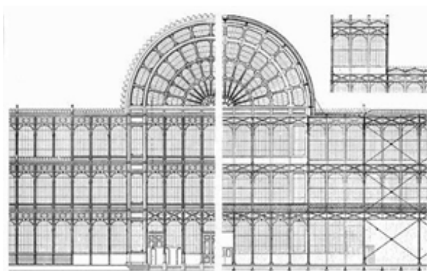
Рис.2. Креслення фасаду Кришталевому палацу.
