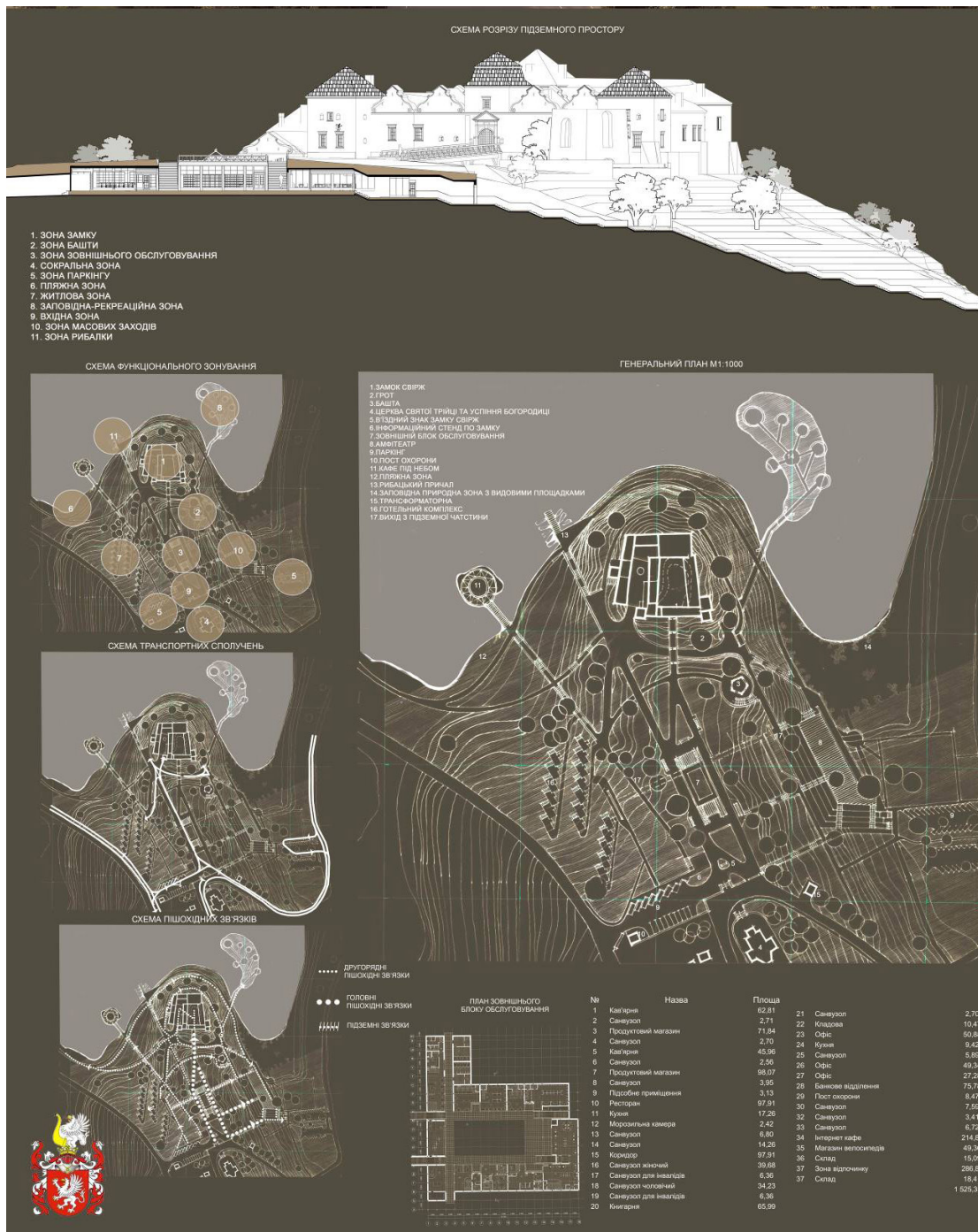
Рис. 13. Матеріали конкурсного проєктного рішення щодо пристосування замку у м. Свірж, Львівської області
