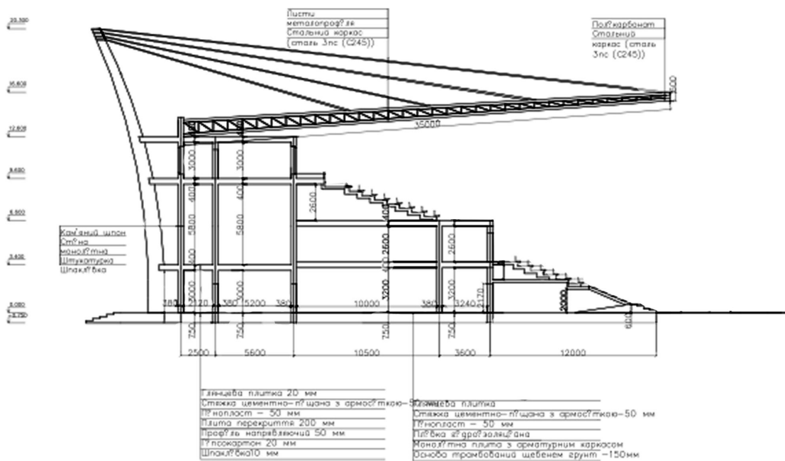
Рис. 14. Влаштування навісів над трибунами стадіону, м. Маріуполь, проектне рішення (автори – М. Чернишева, К. Коробко, 2020 рік)
