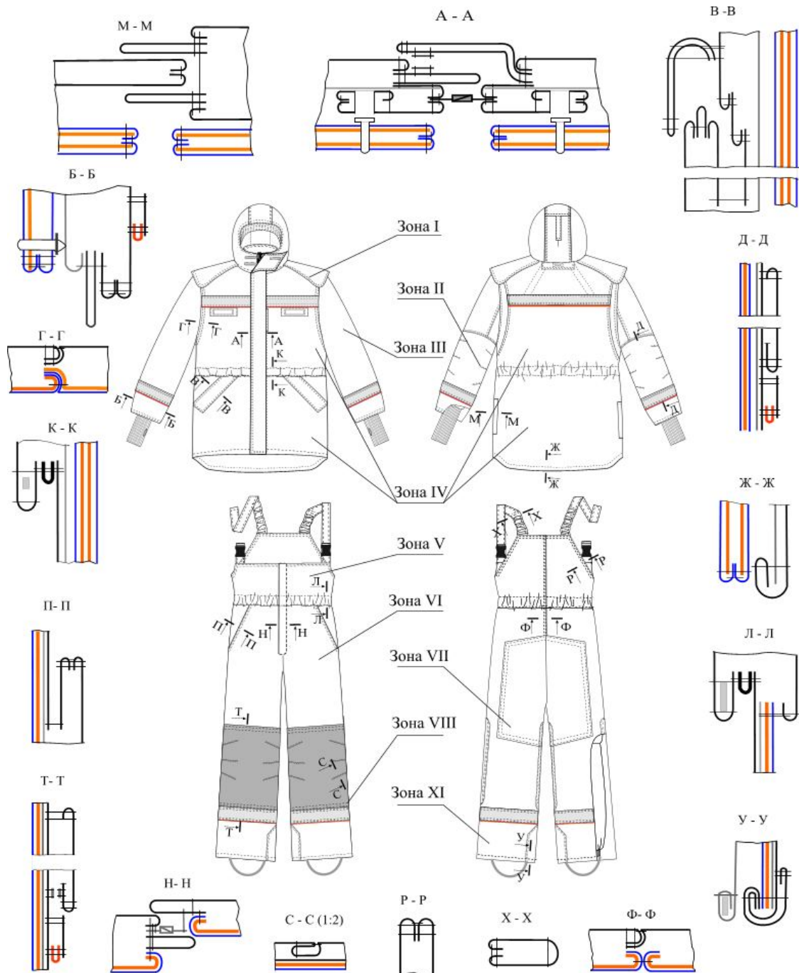
Рис.1. Конструктивно-технологічне рішення комплексу аварійно-рятувального спеціального одягу «ТАРК – 12» та схеми обробки основних вузлів із зональним розташуванням пакетів
